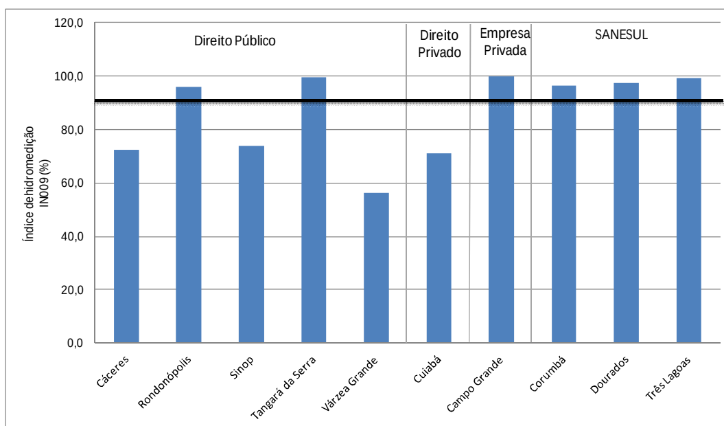
Figura 17 – Índice de hidromedição
