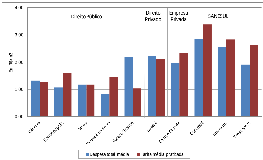
Figura 18 - Tarifa média de água e Despesa média com serviços (R$/m³)
