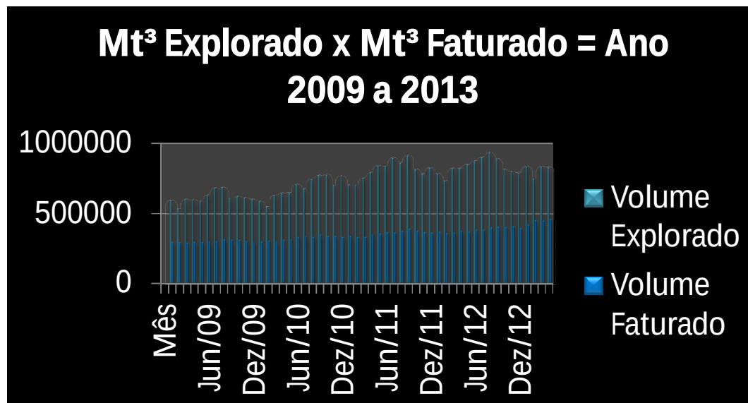
Gráfico 5: Correlação entre as quantidades em m 3 de Água Explorada x Faturada
