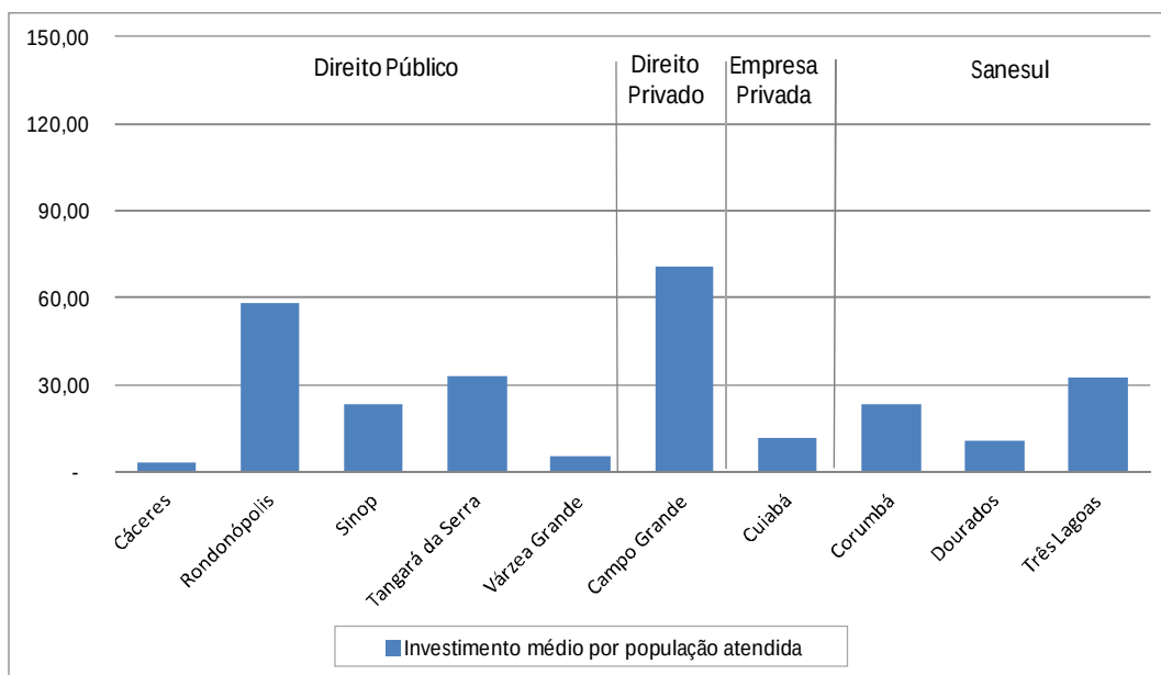
Figura 22 - Investimento em água/população atendida - média de 2007-11
