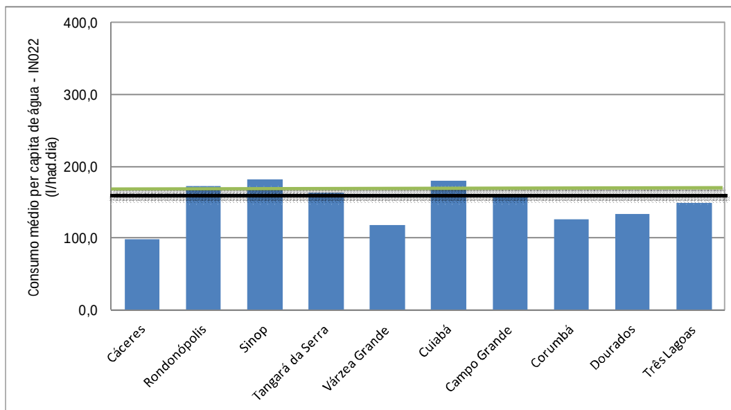
Figura 16 – Consumo médio per capita de água
